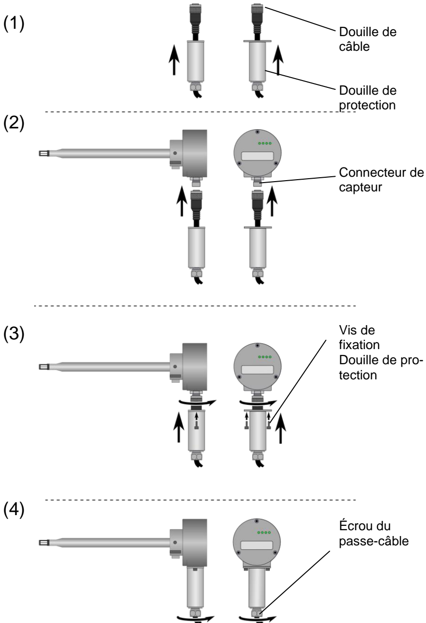
Figure 6-1 Montage câble de raccordement avec douille de protection
