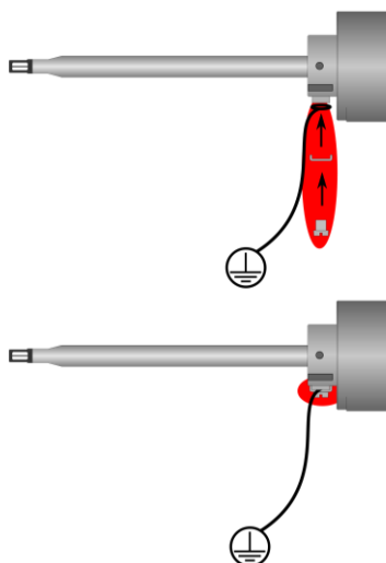
Illustration 5-2 mises à la terre (rouge) capteur compact
