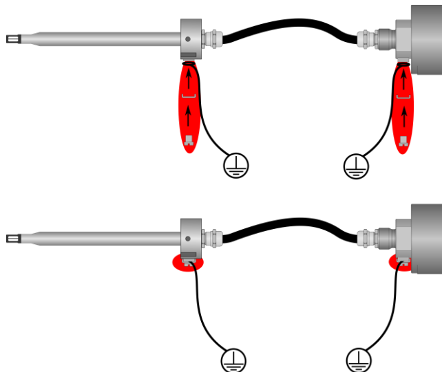
Illustration 5-1 mises à la terre (rouge) version décalée
