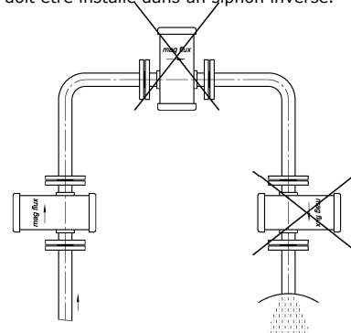
Figure 5 Montage dans des conduites montantes et descendantes
