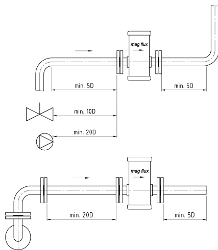
Figure 3 Montage entre coudes de tuyau, vannes et pompes
