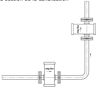
Figure 2 Montage sur canalisations horizontales et verticales
