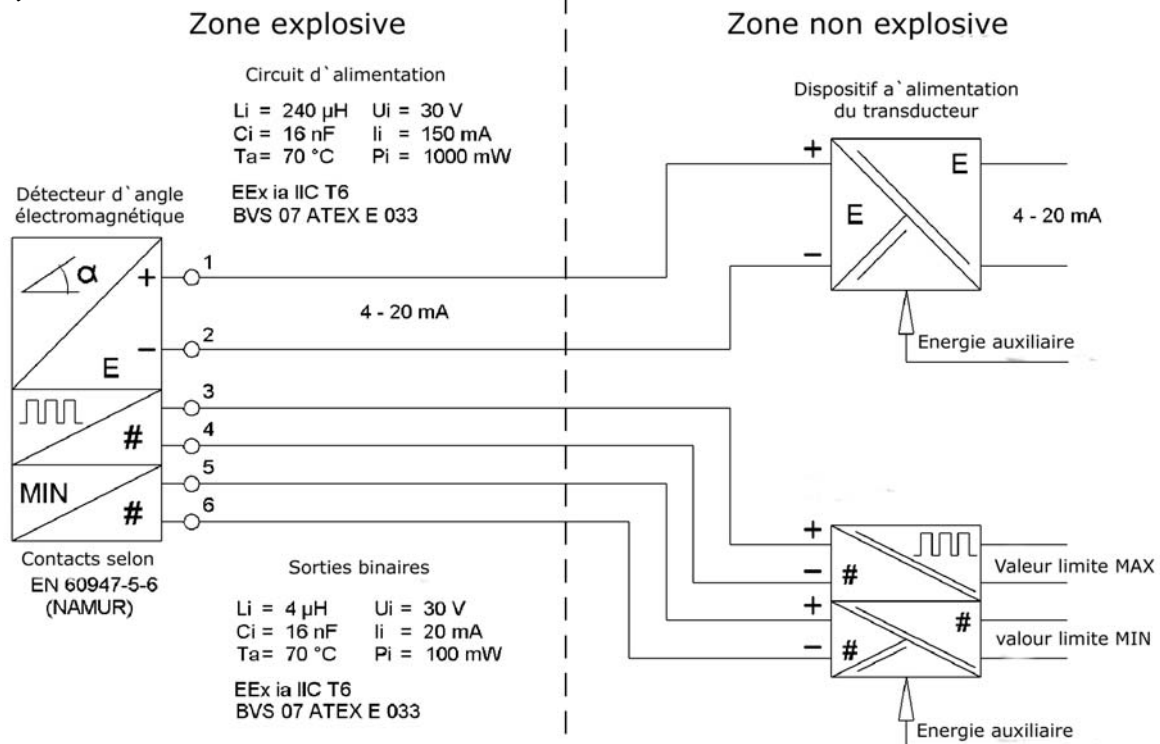
b) Schéma de raccordement du transducteur MEM à sortie 4-20mA et 2 contacts de valeur limite
