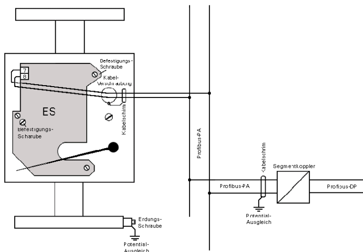
Figure 4 Branchement électrique du MEM-PPA (sur le PROFIBUS-PA)
