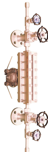
fig.4: STG-IL
