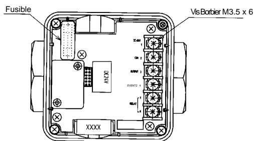
Modèle alimentation 24Vcc
