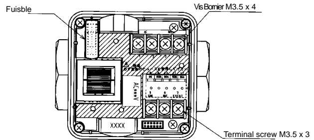
Modèle alimentation CA
