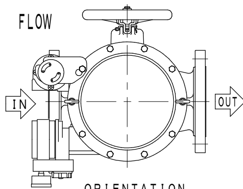
ORIENTATION 配管取付姿勢 No. 1
